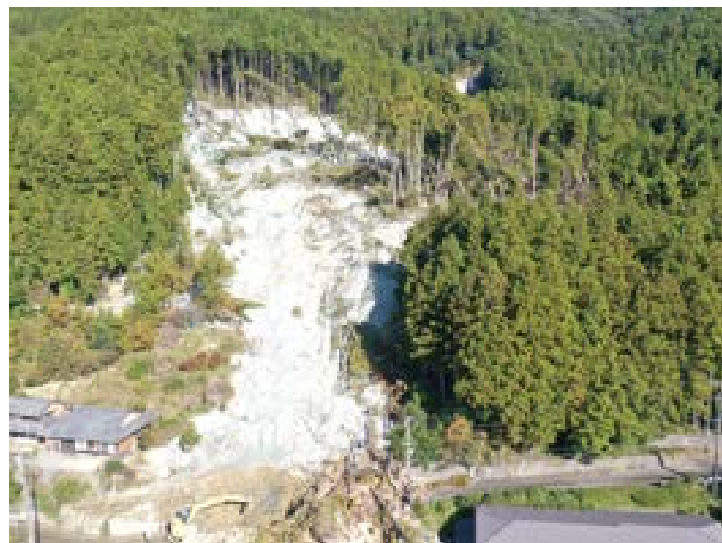
10月10日に災害発生。1ヵ月の11月9日から5日間で14,000m 2 の応急工事が完了
